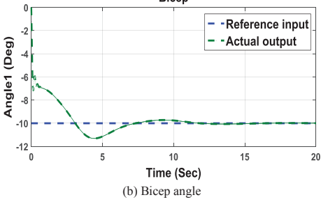
(b) Bicep angle
